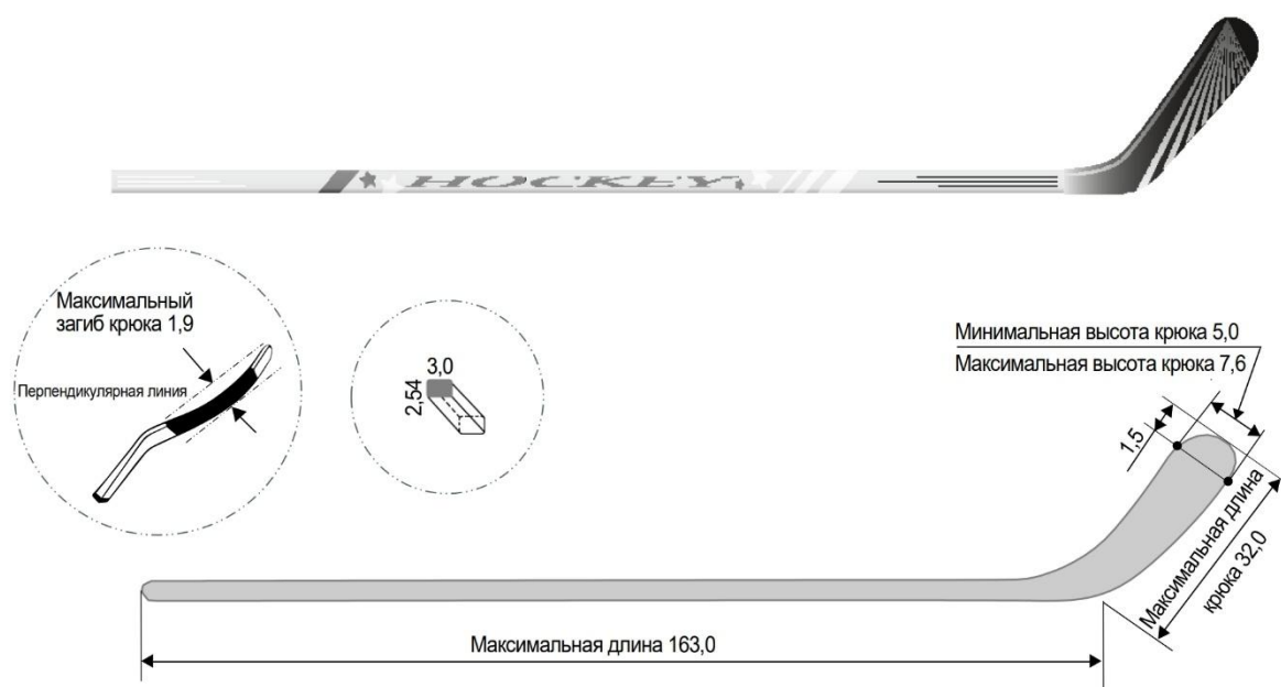
Рисунок 27. Клюшка игрока
